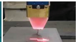
〈용접 갭 보상 시스템〉
