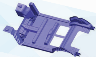
〈 일체형 하부 언더바디 구조 예시 〉
