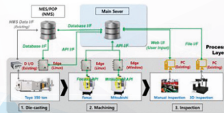
〈 AI기반 공정 지능화 다이캐스팅 공정 〉
